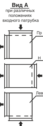
Примеры размещения вентилятора ВРП ДУ (пристенное исполнение)
