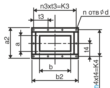
Рис. 2: патрубок входа охлаждающего воздуха
