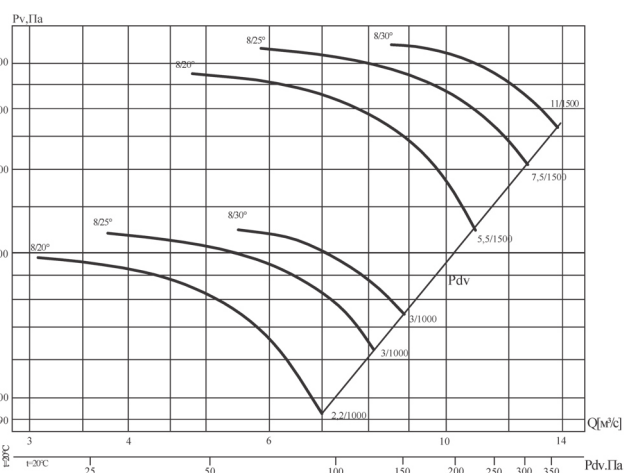
Аэродинамические характеристики вентилятора B' 13-284-8/(20°, 25°, 30°)-9
