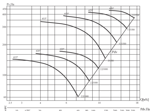
Аэродинамические характеристики вентилятора В' 13-284-4/(15°, 20°, 25°, 30°)-10
