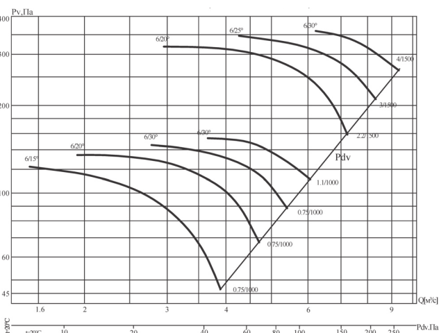
Аэродинамические характеристики вентилятора В' 13-284-6/(15°, 20°, 25°, 30°)-8
