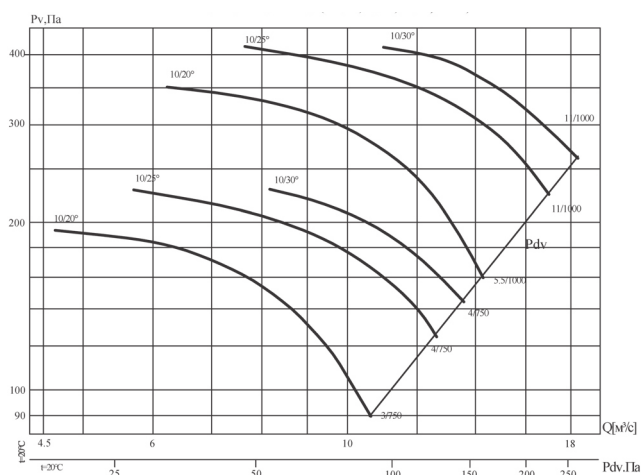
Аэродинамические характеристики вентилятора В' 13-284-10/(20°,25°,30°)-11,2
