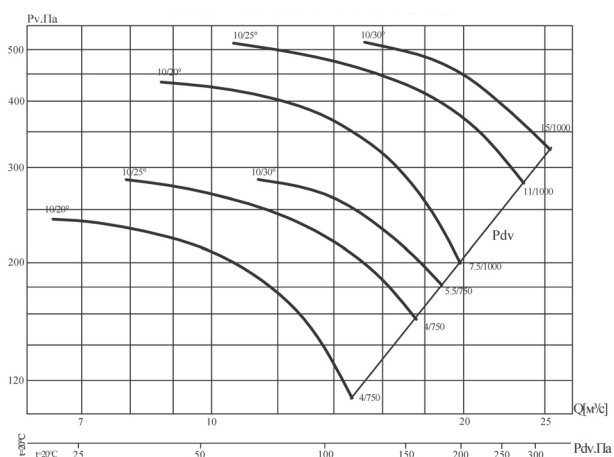
Аэродинамические характеристики вентилятора B' 13-284-10/(20°, 25°, 30°)-12,5
