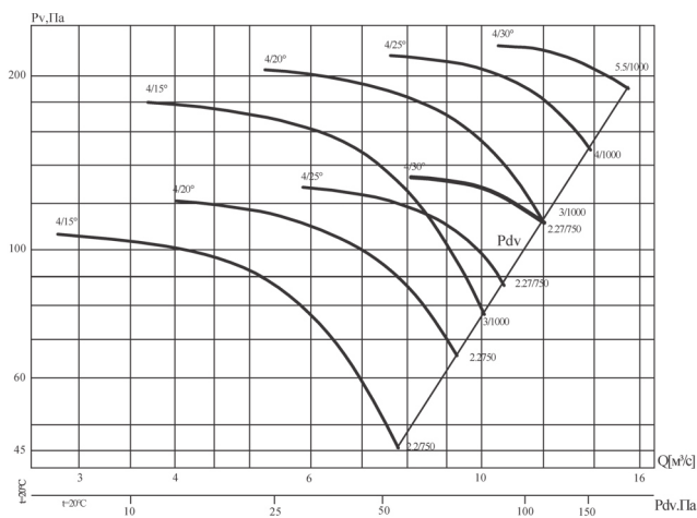
Аэродинамические характеристики вентилятора В' 13-284-4/(15°, 20°, 25°, 30°)-11,2
