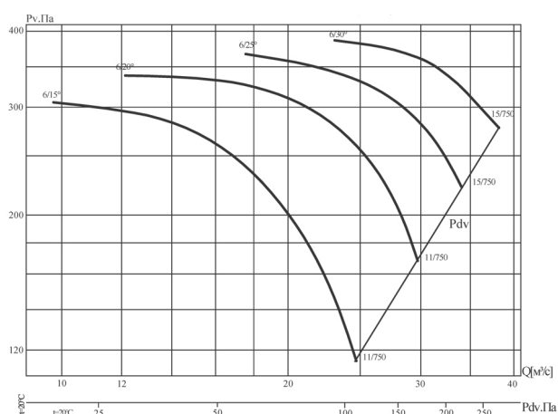
Аэродинамические характеристики вентилятора B' 13-284-6/(15°, 20°, 25°, 30°)-16
