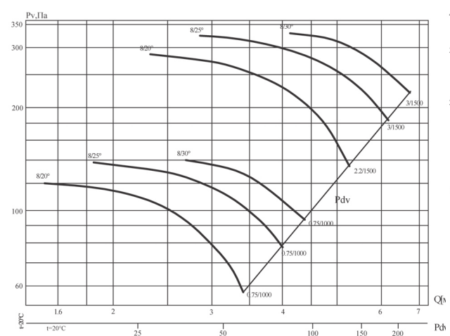
Аэродинамические характеристики вентилятора В' 13-284-8/(20°, 25°, 30°)-7,1
