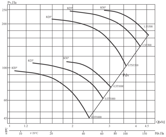
Аэродинамические характеристики вентилятора В' 13-284-8/(20°, 25°, 30°)-6,3
