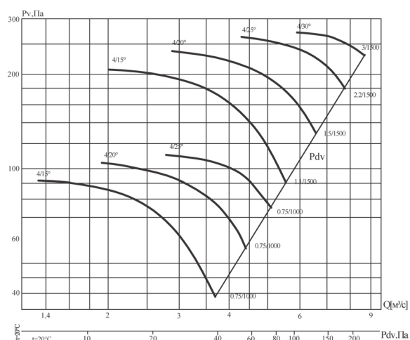
Аэродинамические характеристики вентилятора В' 13-284-4/(15°, 20°, 25°, 30°)-8
