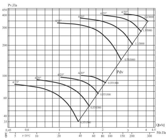
Аэродинамические характеристики вентилятора В' 13-284-4/(15°,20°,25°,30°)-5
