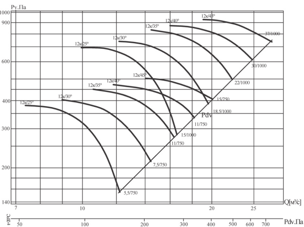
Аэродинамические характеристики вентилятора В' 13-284-12к/(25°, 30°, 35°, 40°, 45°)-12,5
