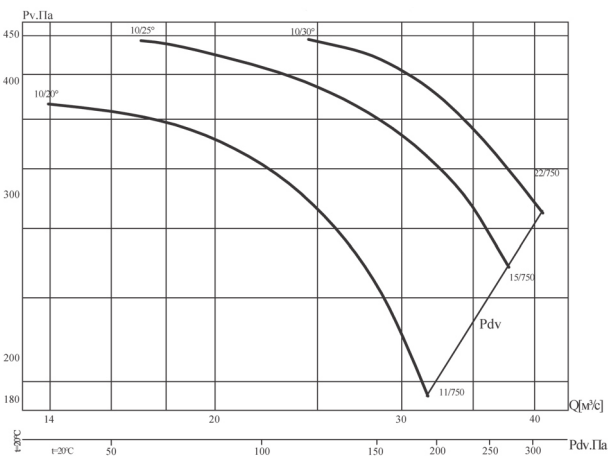
Аэродинамические характеристики вентилятора B' 13-284-10/(20°, 25°, 30°)-16
