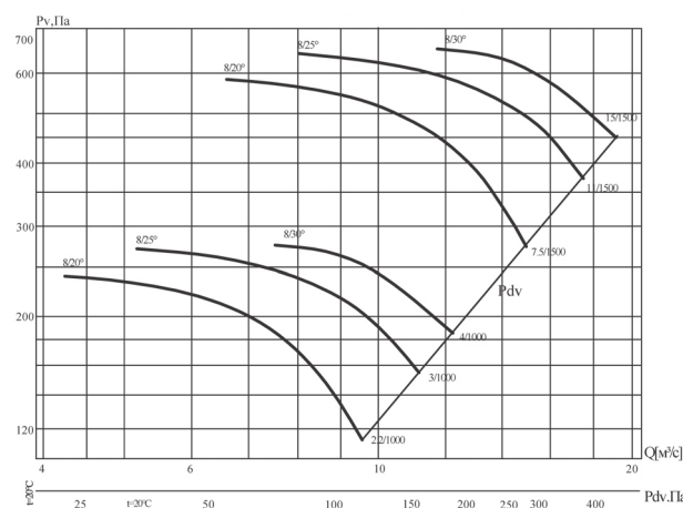
Аэродинамические характеристики вентилятора В' 13-284-8/(20°, 25°, 30°)-10
