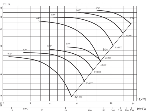
Аэродинамические характеристики вентилятора B' 13-284-6/(15°, 20°, 25°, 30°)-9
