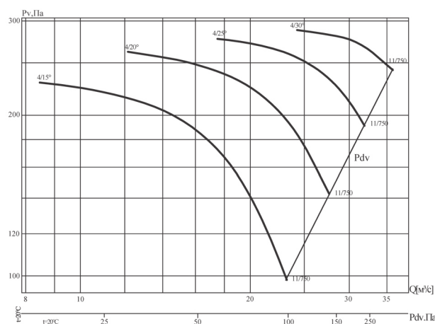
Аэродинамические характеристики вентилятора B' 13-284-4/(15°, 20°, 25°, 30°)-16
