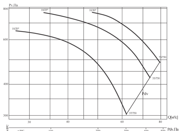
Аэродинамические характеристики вентилятора В' 13-284-10/(20°, 25°, 30°)-20
