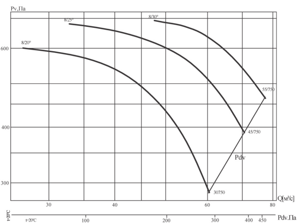
Аэродинамические характеристики вентилятора В' 13-284-8/(20°, 25°, 30°)-20
