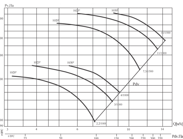
Аэродинамические характеристики вентилятора B' 13-284-10/(20°, 25°, 30°)-9
