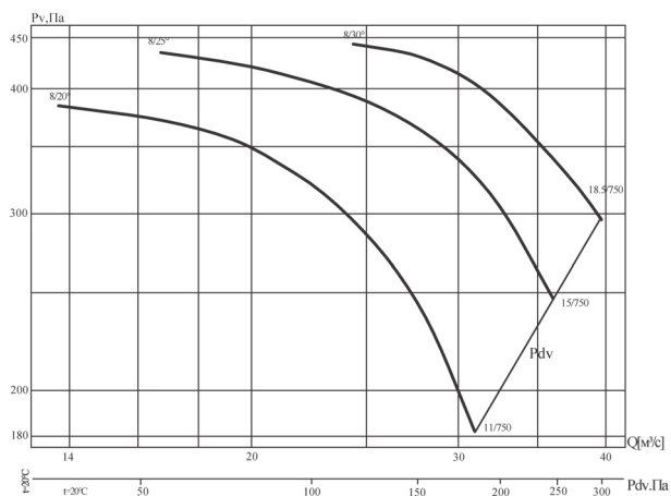
Аэродинамические характеристики вентилятора B' 13-284-8/(20°, 25°, 30°)-16
