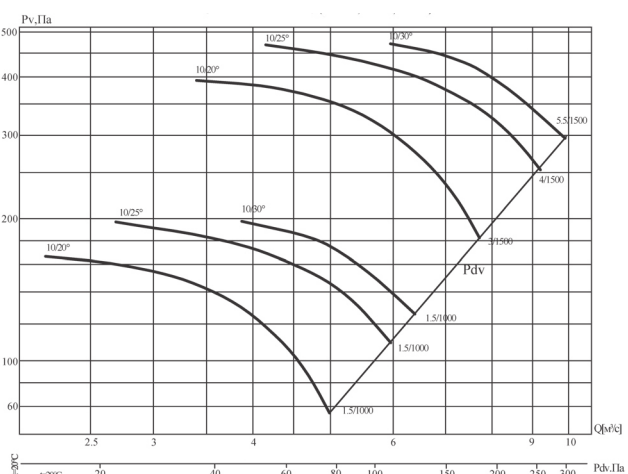
Аэродинамические характеристики вентилятора B' 13-284-10/(20°, 25°, 30°)-8
