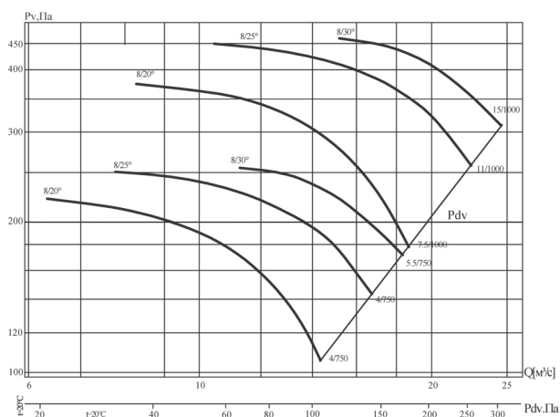
Аэродинамические характеристики вентилятора B' 13-284-8/(20°, 25°, 30°)-12,5
