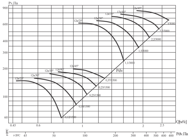
Аэродинамические характеристики вентилятора В' 13-284-12к/(25°, 30°, 35°, 40°, 45°)-4
