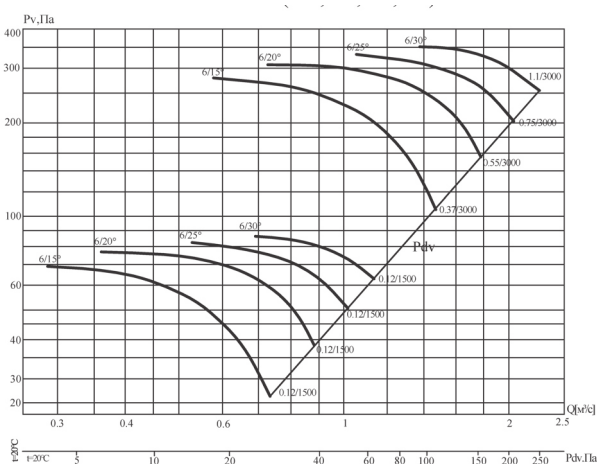
Аэродинамические характеристики вентилятора В' 13-284-6/(15°,20°,25°,30°)-4
