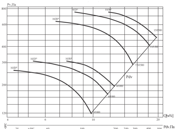
Аэродинамические характеристики вентилятора В' 13-284-10/(20°, 25°, 30°)-10
