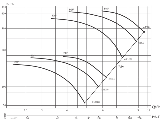
Аэродинамические характеристики вентилятора B' 13-284-8/(20°, 25°, 30°)-8
