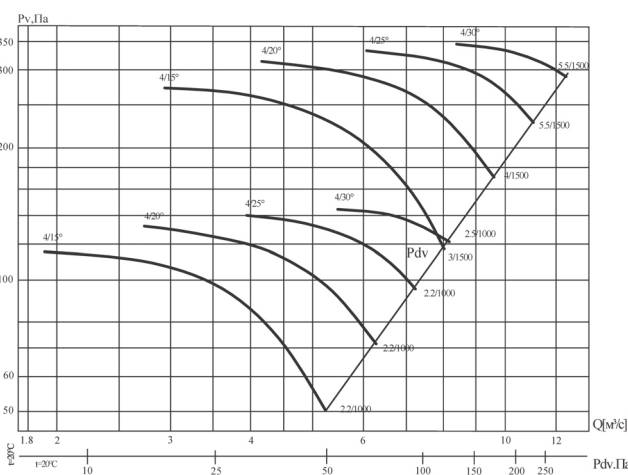
Аэродинамические характеристики вентилятора B' 13-284-4/(15°, 20°, 25°, 30°)-9
